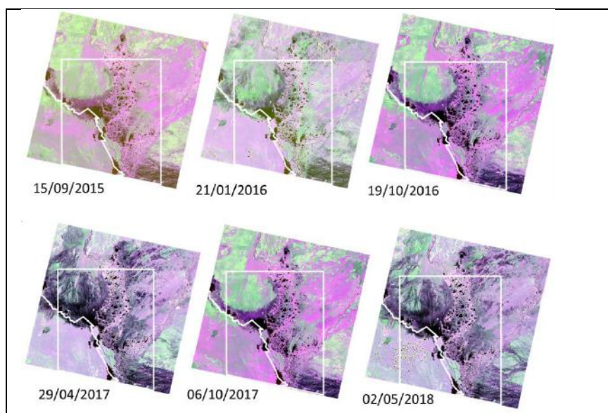
Figura 3 – Composição R(NDWI)G(5)B(6).
